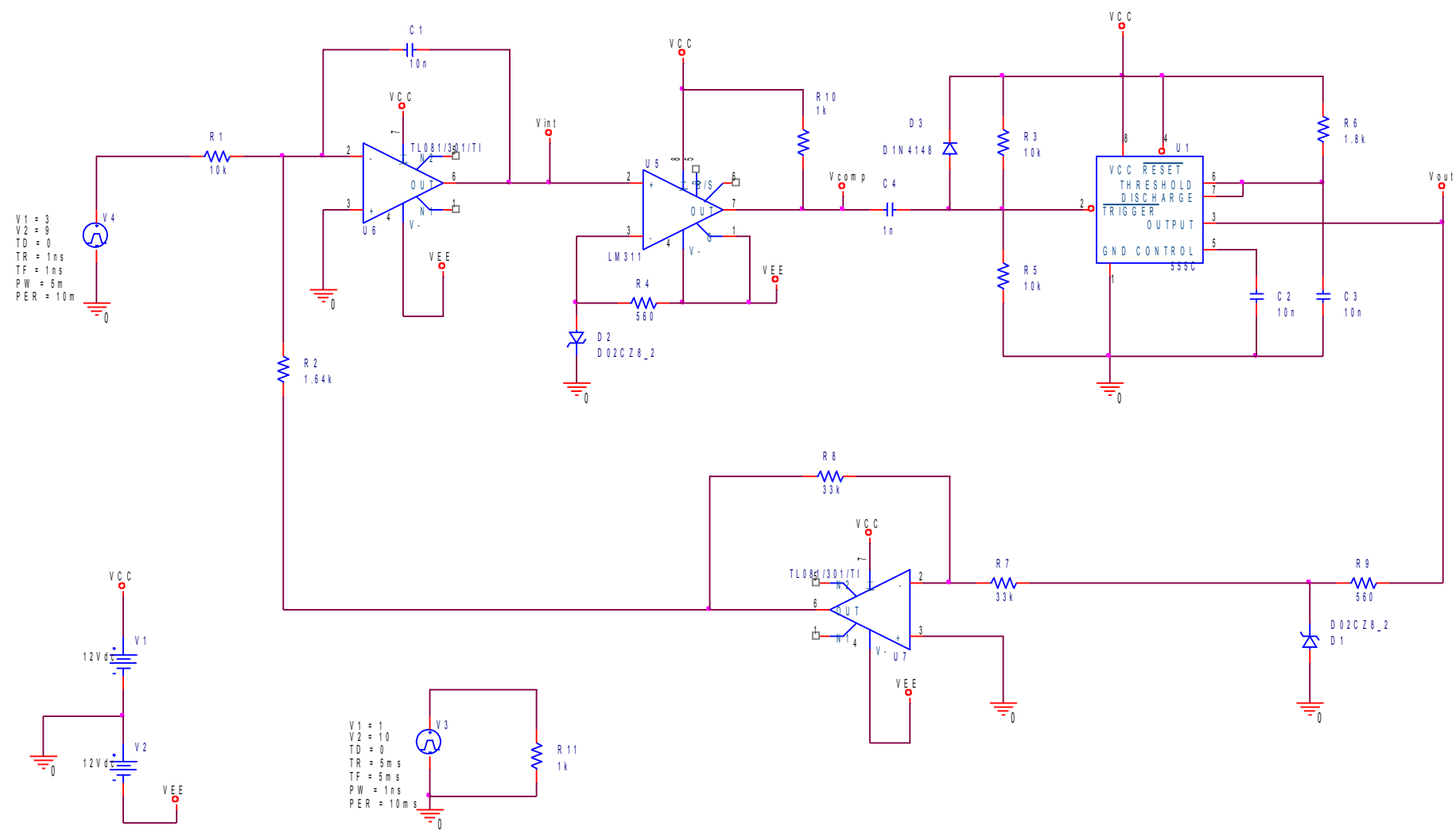
Schema generale del convertitore Tensione-Frequenza.
